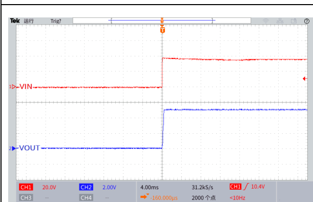
图 26.上电波形图
