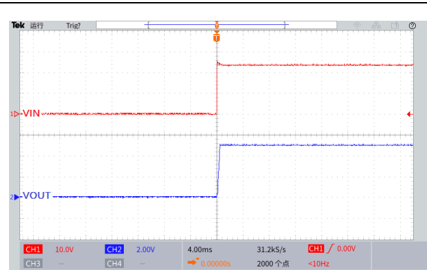
图 25.上电波形图
