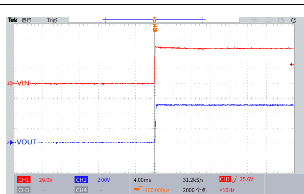
图 27.上电波形图
