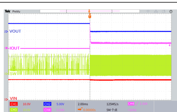
图 29.输出短路波形
