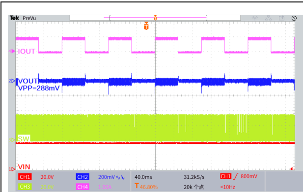
图 28.瞬态负载响应波形
