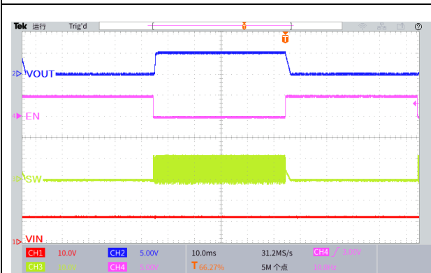
图 30.EN 引脚开关机波形
