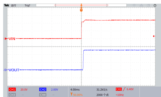
图 25.上电波形图
