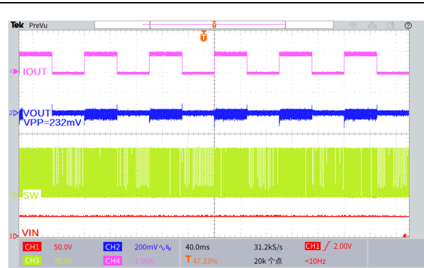
图 29.瞬态负载响应波形
