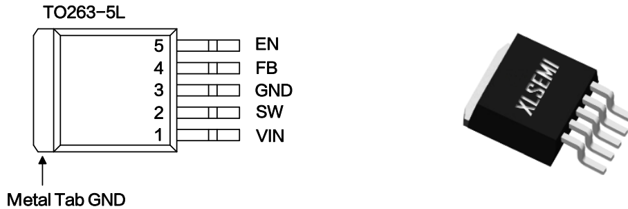
图 2. XL2576HVS 引脚配置
