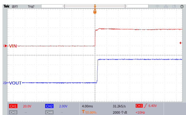
图 24.上电波形图
