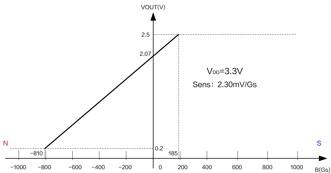
图 5.XL42W 输出特性曲线 ( V_{DD} = 3.3V )
