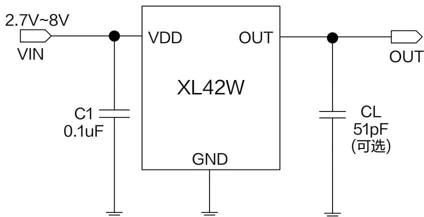
图 1.XL42W 典型应用示意图
