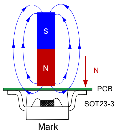
图 4.XL42W 应用图
