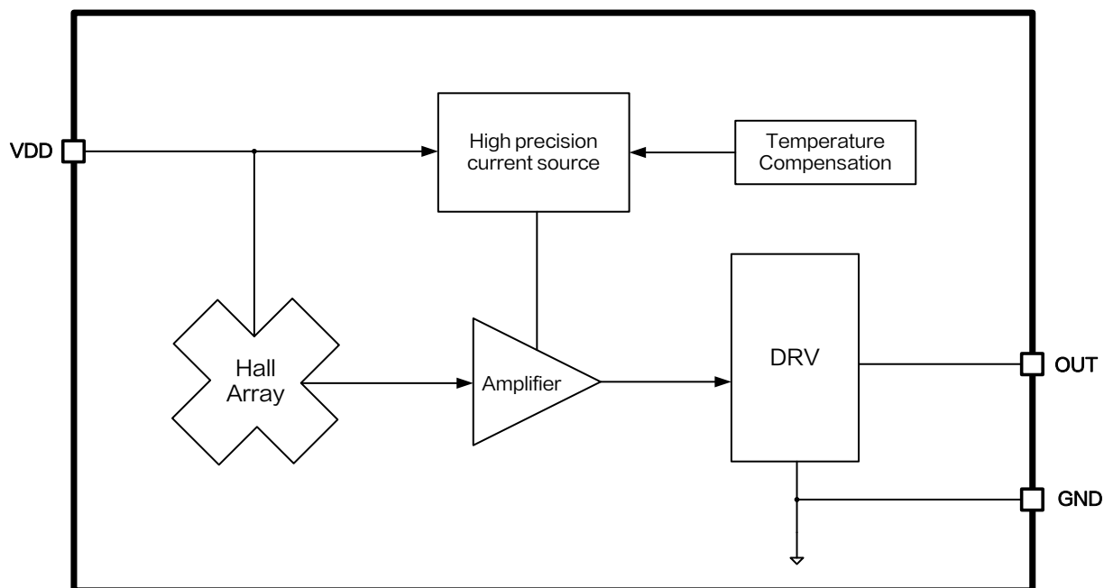
图 3.XL42W 功能方框图
