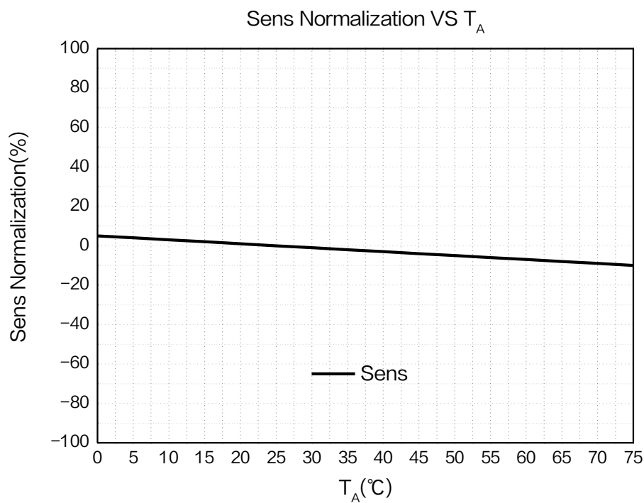
图 7.XL42W 灵敏度随温度变化曲线 ( V_{DD} = 3.3V )
