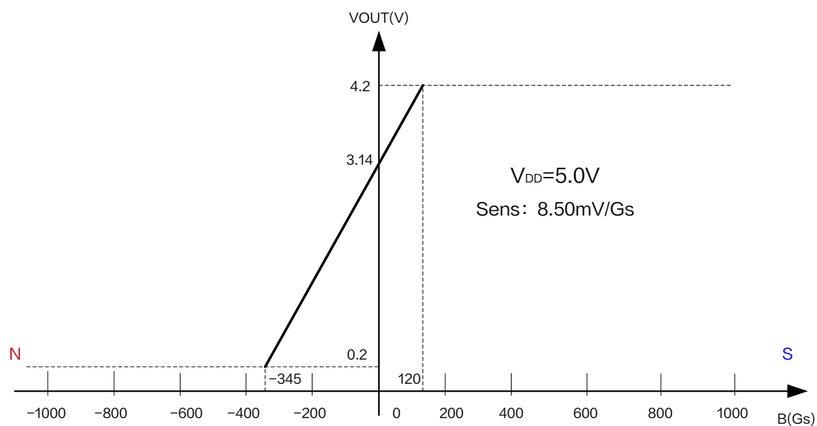
图 6.XL42W 输出特性曲线 ( V_{DD} = 5.0V )
