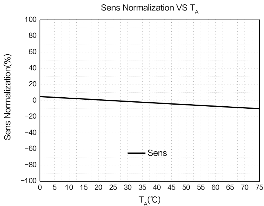
图 7.XL42Y 灵敏度随温度变化曲线 ( V_{DD} = 3.3V )
