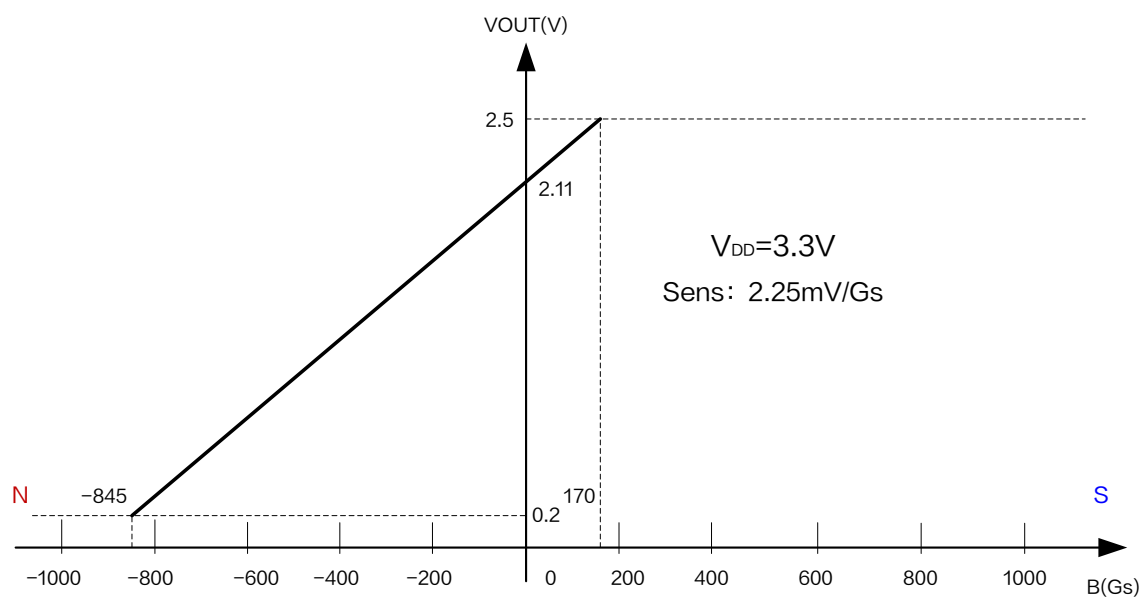
图 5.XL42Y 输出特性曲线 ( V_{DD} = 3.3\text{V} )
