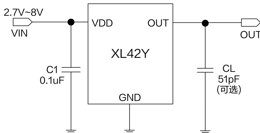
图 1.XL42Y 典型应用示意图
