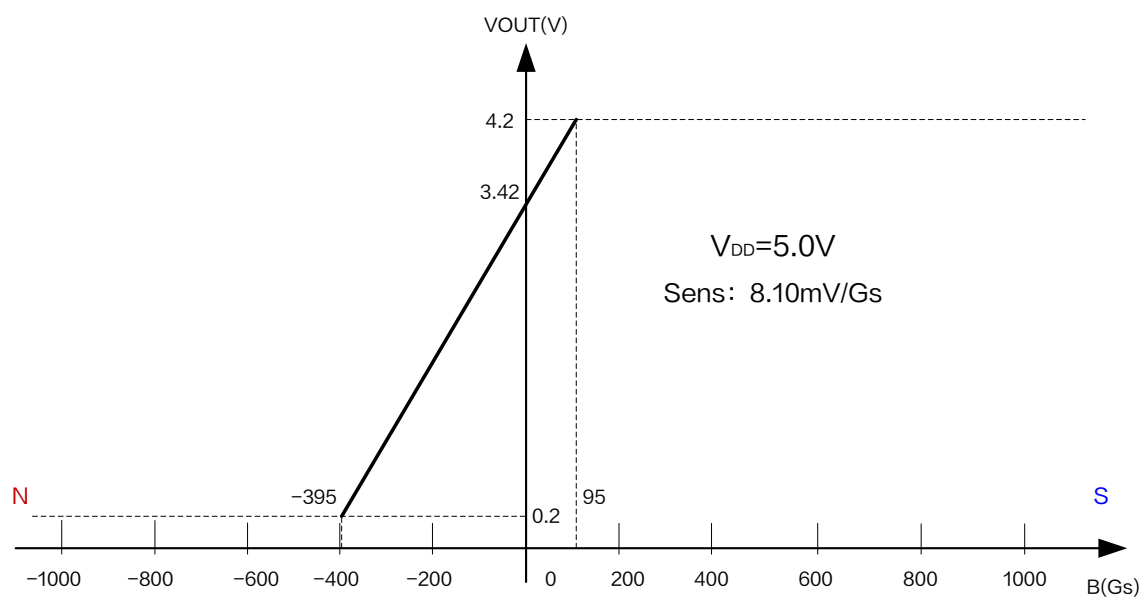
图 6.XL42Y 输出特性曲线 ( V_{DD} = 5.0V )
