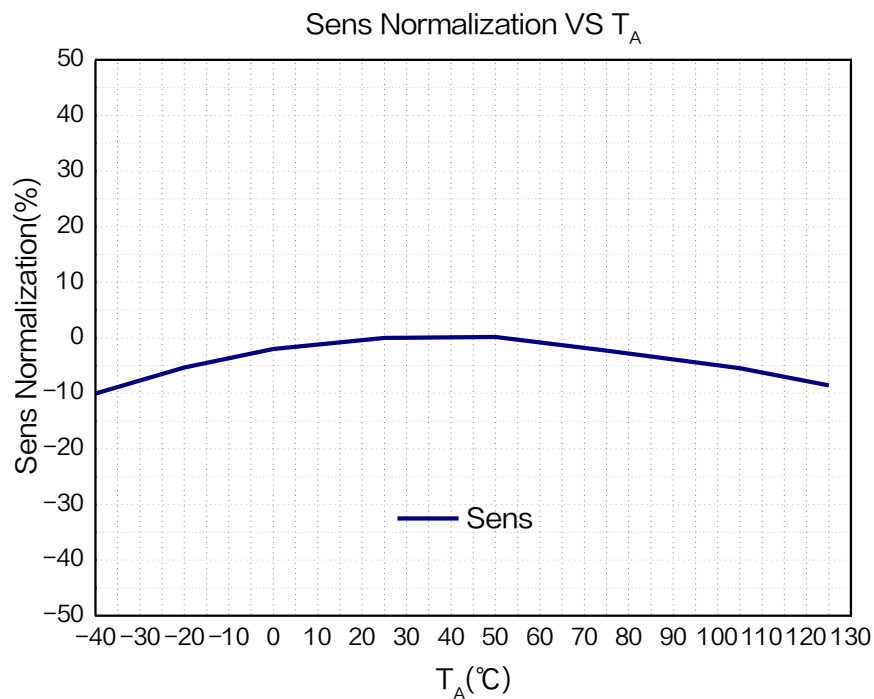
图 8.XL47E 灵敏度随温度变化曲线 ( V_{DD} = 5.0V )
