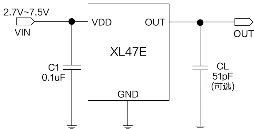
图 1.XL47E 典型应用示意图
