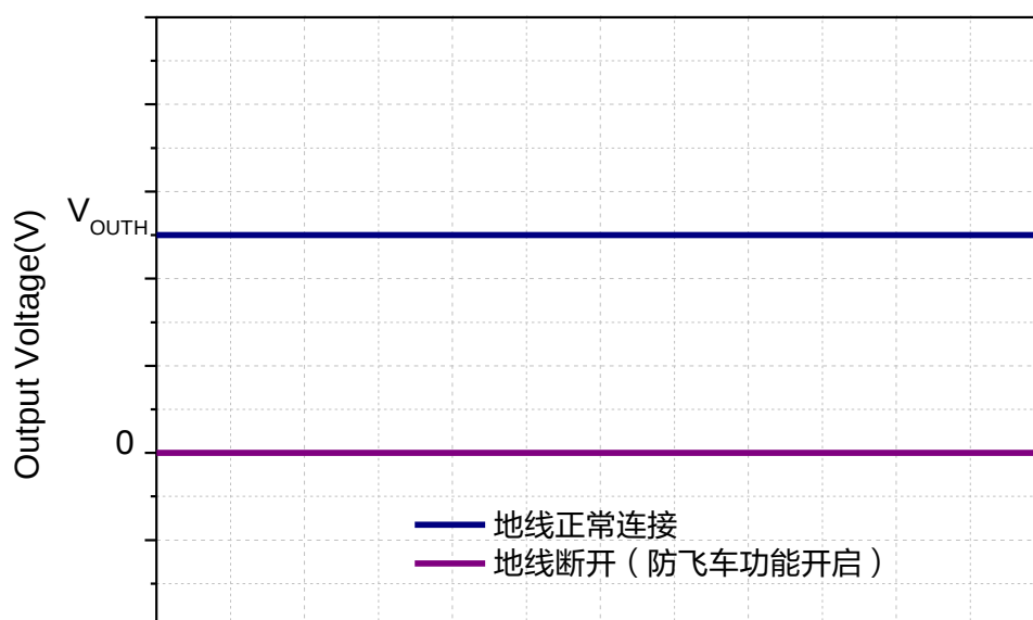
图 7.XL47E 防飞车功能特性曲线 ( V_{DD} = 5.0V )
