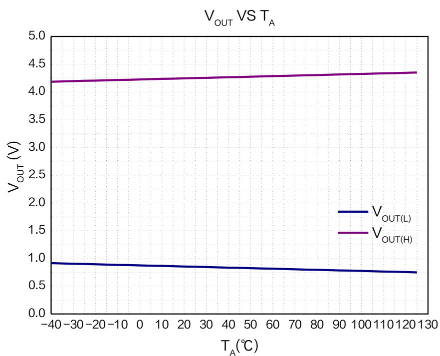
图 10.XL47E 输出高/低电平温度特性曲线 ( V_{DD} = 5.0V )
