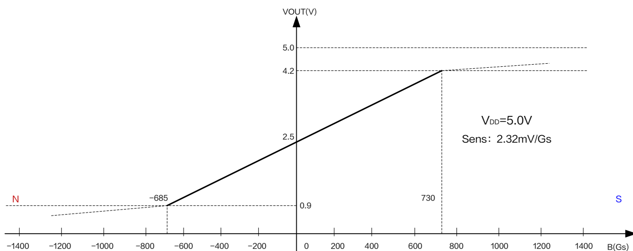
图 5.XL47E 输出特性曲线 ( V_{DD} = 5.0\text{V} )
