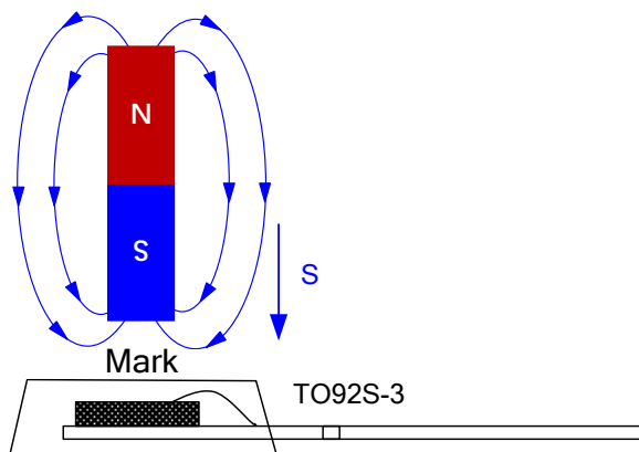
图 4.XL47E 应用图
