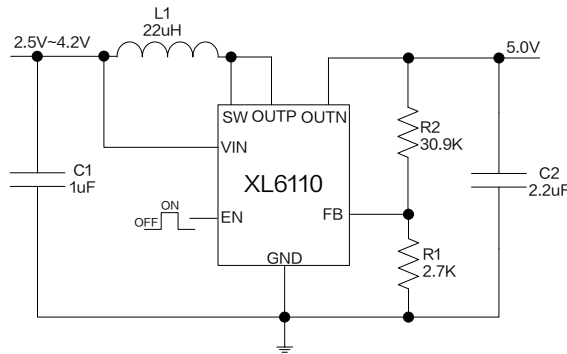
图 4. XL6110 系统参数测量电路及效率曲线图 ( V_{OUT}=5.0V )
