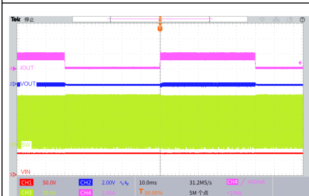
图 24.瞬态负载响应波形 ( V_{IN}=72V , V_{OUT}=12V , I_{OUT}=0.1 至 0.8A )
