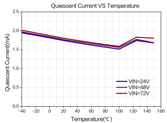
图 11.静态电流温度系数曲线图
