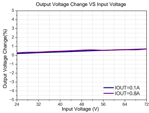
图 8.线性调整率曲线图
