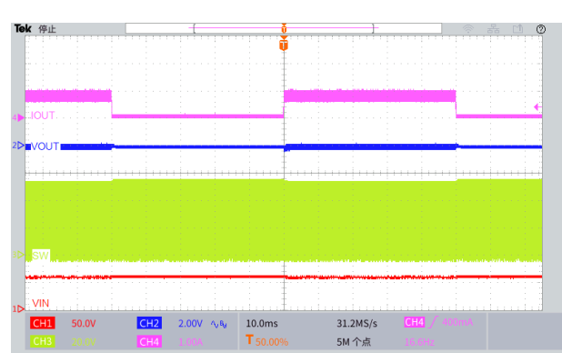
图 23.瞬态负载响应波形 ( V_{IN}=60V , V_{OUT}=12V , I_{OUT}=0.1 至 0.8A )
