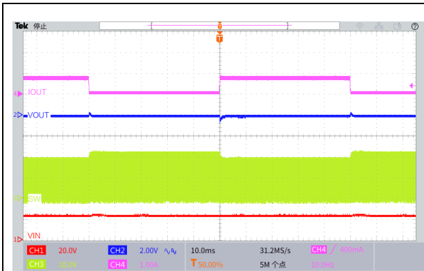
图 20.瞬态负载响应波形 ( V_{IN}=24V , V_{OUT}=12V , I_{OUT}=0.1 至 0.8A )
