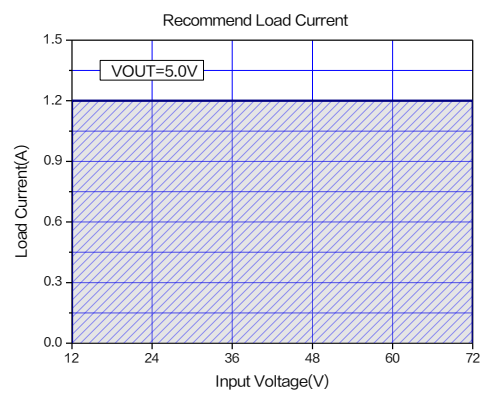
图 13.最大输出电流 ( V_{OUT}=5.0V , T_A=25^{\circ}C )
