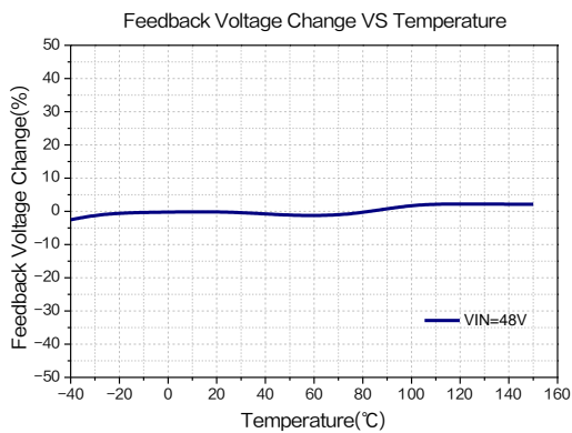
图 12.反馈电压温度系数曲线图
