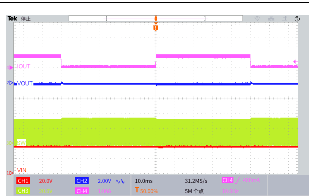
图 21.瞬态负载响应波形 ( V_{IN}=36V , V_{OUT}=12V , I_{OUT}=0.1 至 0.8A )
