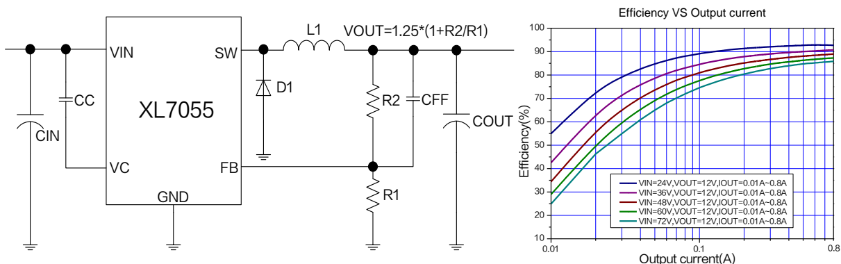
图1.XL7055典型应用示意图和转换效率曲线
