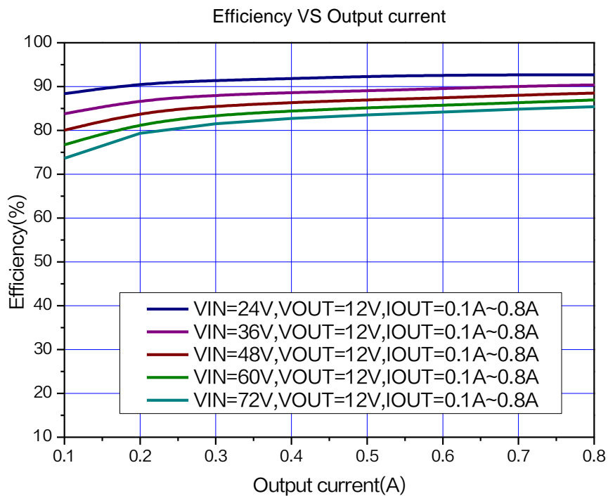
图 7.XL7055 系统效率曲线 ( V_{OUT}=12V )
