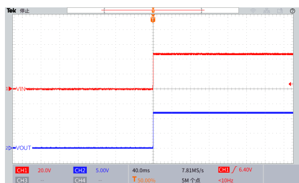
图 17.上电波形图 ( V_{IN}=48V , V_{OUT}=12V , I_{OUT}=0.1A )
