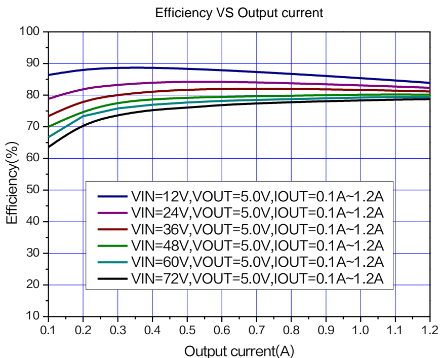
图 5.XL7055 系统效率曲线 ( V_{OUT}=5.0V )
