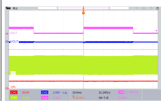
图 22.瞬态负载响应波形 ( V_{IN}=48V , V_{OUT}=12V , I_{OUT}=0.1 至 0.8A )
