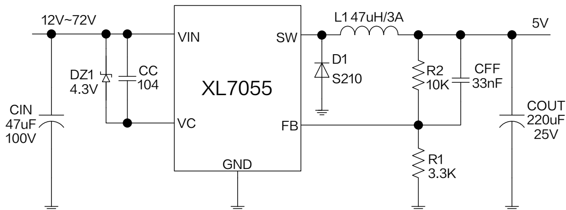
图 4.XL7055 系统参数测量电路 ( V_{IN}=12V\sim 72V , V_{OUT}=5V , I_{OUT}=0\sim 1.2A )
