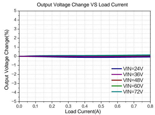
图 9.负载调整率曲线图
