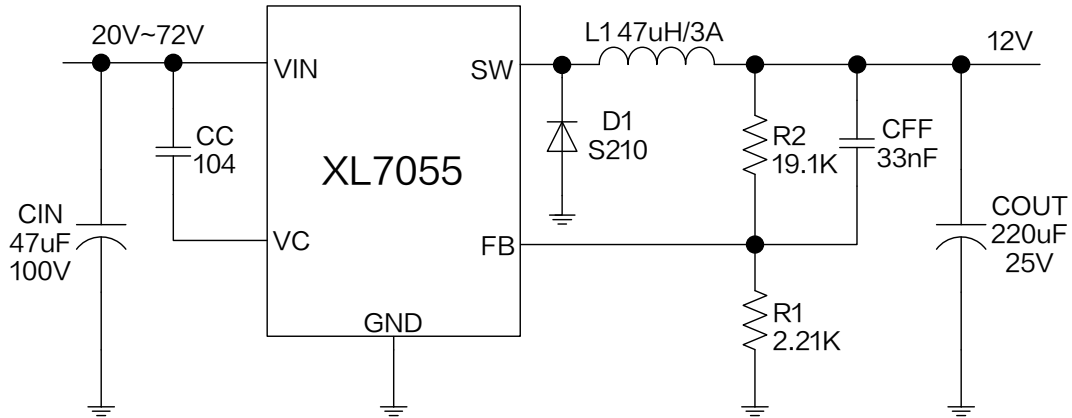
图 6.XL7055 系统参数测量电路 ( V_{IN}=20V\sim 72V, V_{OUT}=12V, I_{OUT}=0\sim 0.8A )
