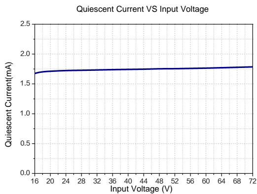
图 10.静态电流曲线图
