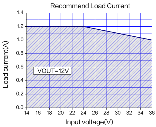
图 18.最大输出电流 ( V OUT =12V, T A =25°C )
