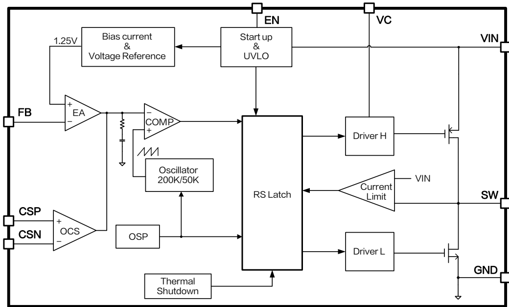
图 3. XL9010 方框图
