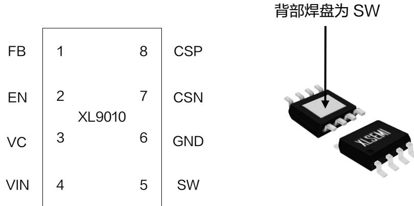
图 2. XL9010 引脚配置
