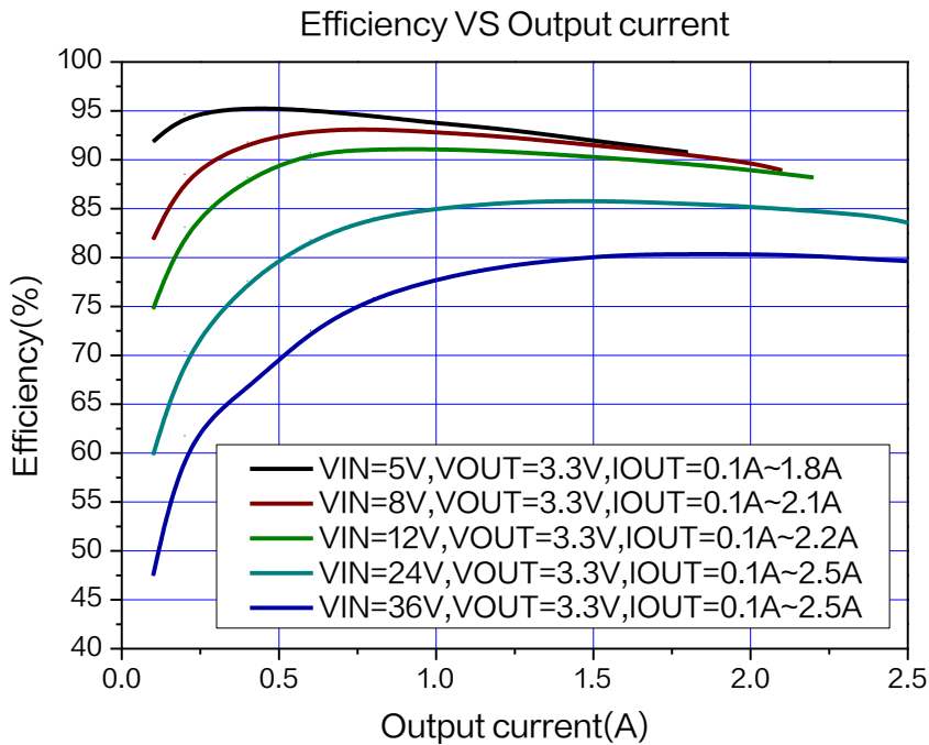
图 5. XL9022 系统效率曲线 ( V_{OUT}=3.3V )
