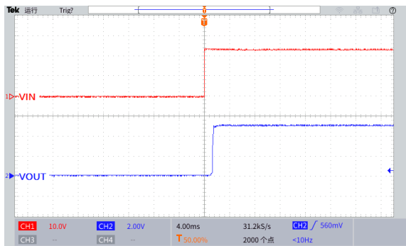
图 24.上电波形图
