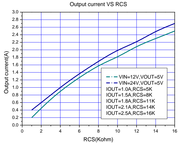
输出电流曲线:
