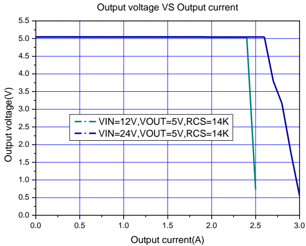
输出恒流曲线:
