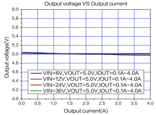
5.0V 输出线性调整率与负载调整率曲线
