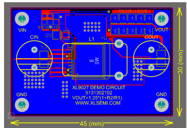
PCB底层截图
