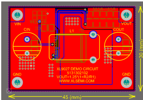
PCB顶层截图
