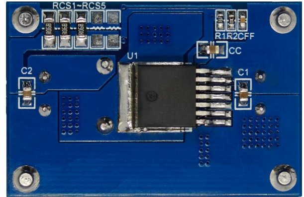
实物图反面
