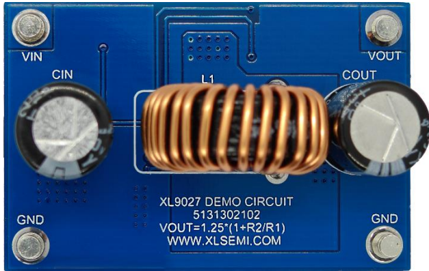
实物图正面
