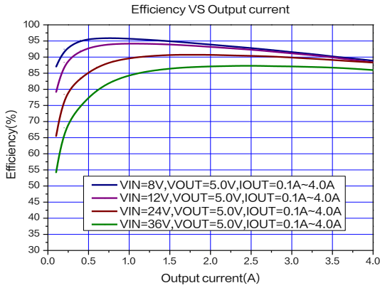
5.0V 输出效率曲线
