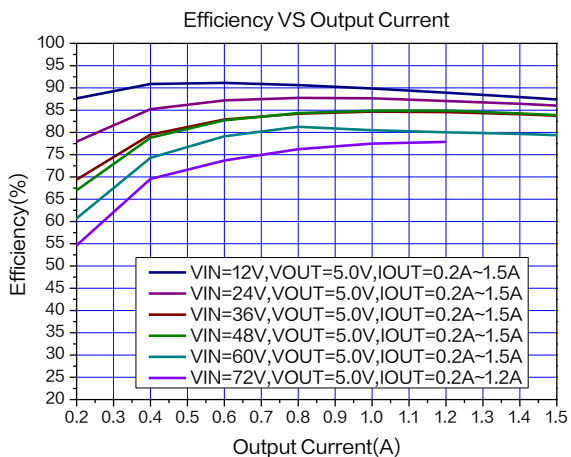
5.0V 输出效率曲线
